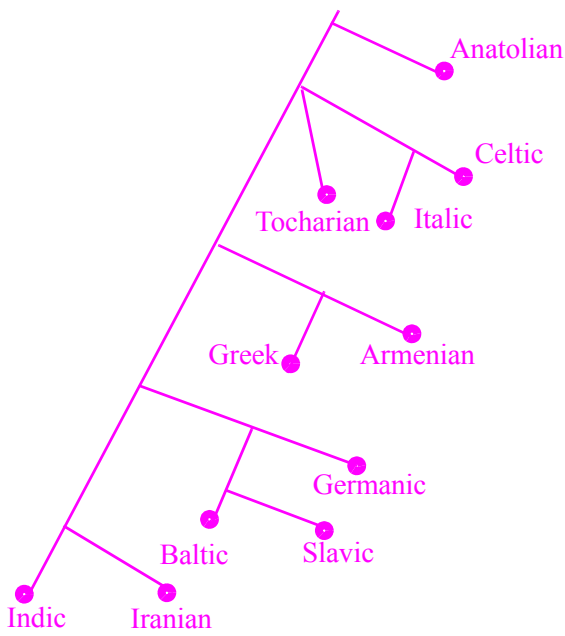
Ringe, (et al ?) Tree
